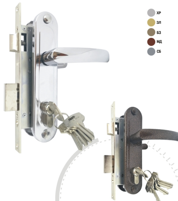
Замок врезной ЗВ7-70 (корпус)
